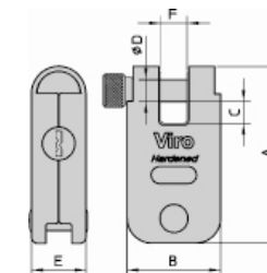
ART. 4239.500
